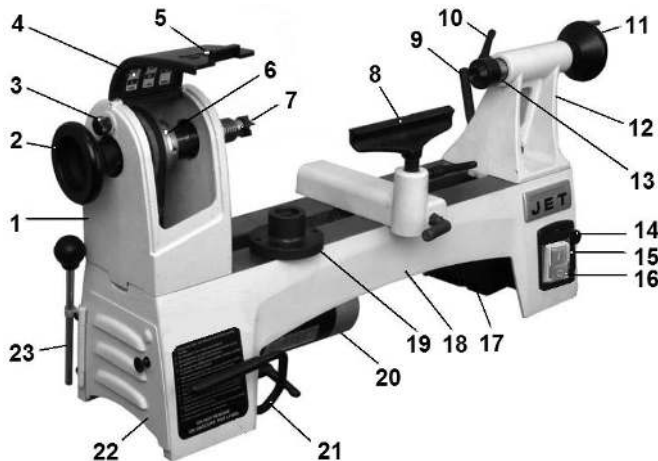
Fig 1 (JWL-1015VS shown)
